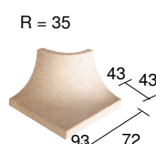
RRE RACCORDO RADIALE ESTERNO - EXTERNAL MITRE (DAV 08 - DAV 31 - GS 84 GSM 17 - PS 14)
