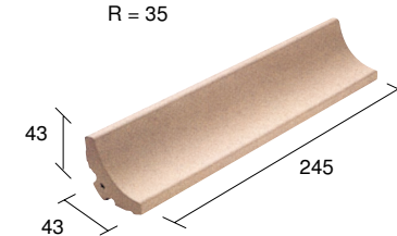
RA RACCORDO A PAVIMENTO FLOOR LEVEL UNION (DAV 08 - DAV 31 - GS 84 GSM 17 - PS 14)
