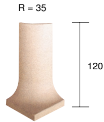
REP RACCORDO ANGOLO ESTERNO EXTERNAL MITRE (DAV 08 - DAV 31 - DAV 46 - DAV 58 GS 84 - GSM 17 - PS 14)
