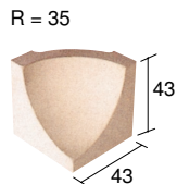
RAA RACCORDO ANGOLO INTERNO - INTERNAL MITRE (DAV 08 - DAV 31 - GS 84 GSM 17 - PS 14)
