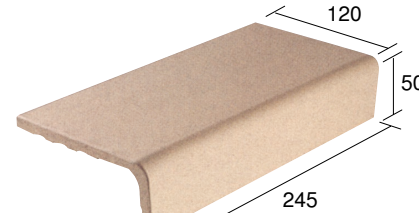
B 60 BORDO ANGOLARE CORNER EDGE (GS 84 - GSM 17 - PS 14)
