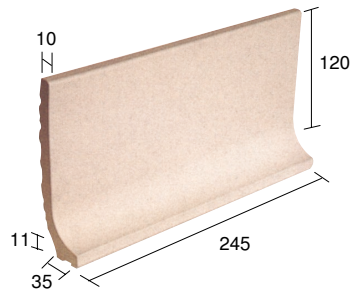
R 42 RACCORDO A PAVIMENTO FLOOR LEVEL UNION (DAV 08 - DAV 31 - DAV 46 - DAV 58 GS 84 - GSM 17 - PS 14)
