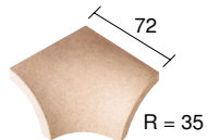
RRI RACCORDO RADIALE INTERNO - INTERNAL MITRE (DAV 08 - DAV 31 - GS 84 GSM 17 - PS 14)
