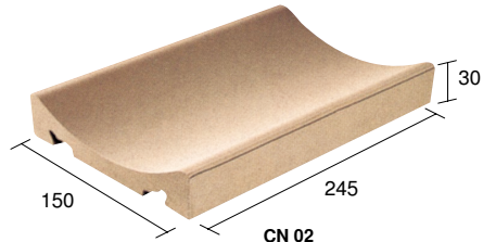
CN 02 CANALETTA - DUCT (GSM 17)
