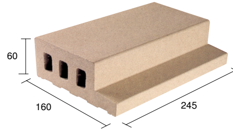
B 59 BORDO REGGIGRIGLIA GRID SUPPORT (DAV 08)
